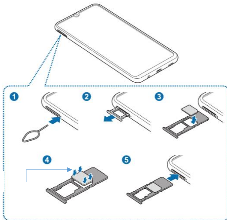
شکل (ج): نحوه ی قرار دادن سیم کارت
